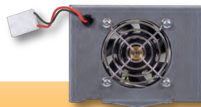
Optional PWB Cooling Fan Available
